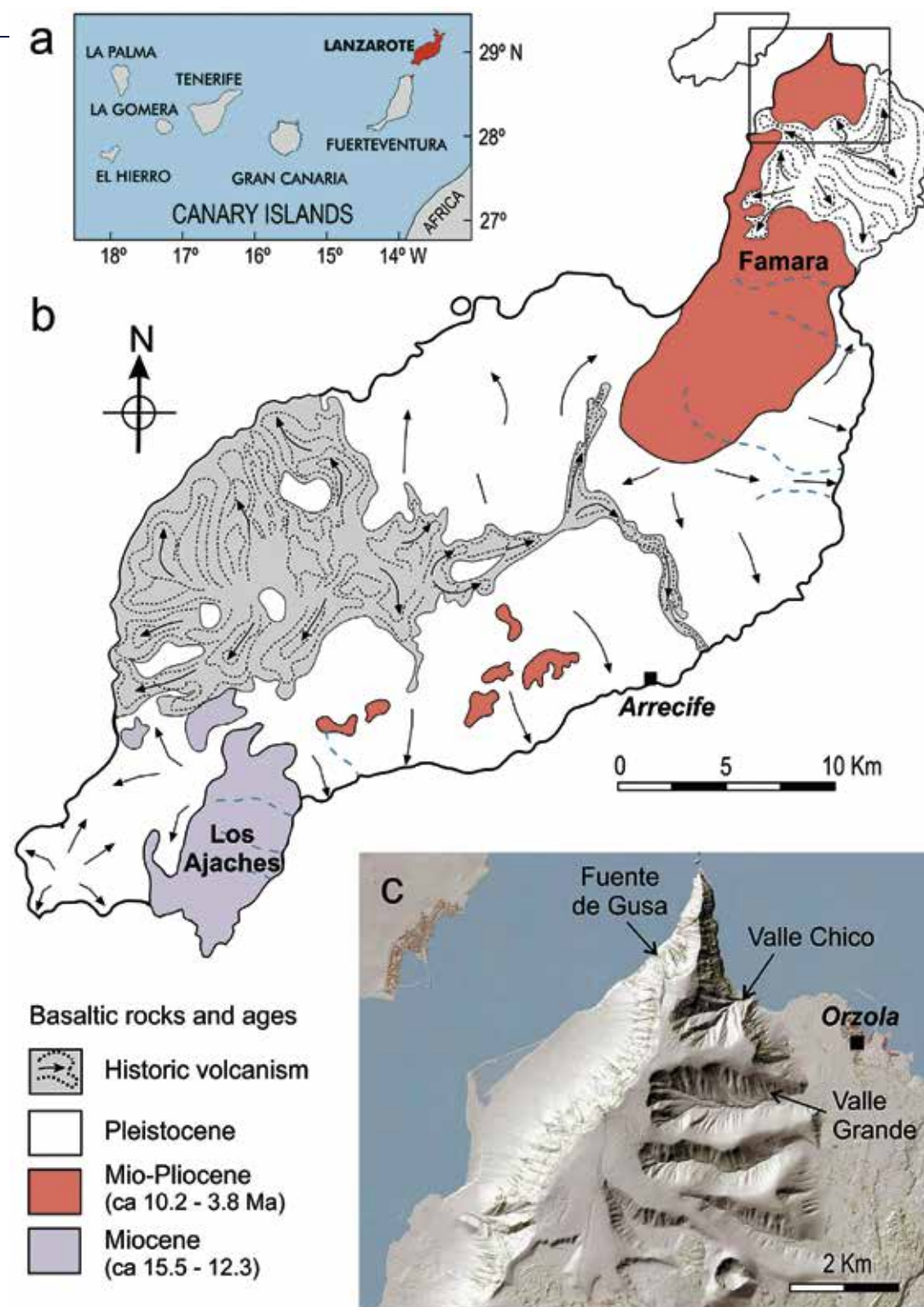
Mapa geológico esquemático de Lanzarote con sus dos edificios volcánicos, Los Ajaches y Famara. Ubicación de los yacimientos fosilíferos (área recuadrada).
